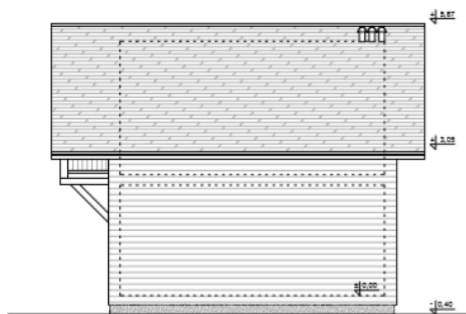
ELEWACJA POŁUDNIOWA
